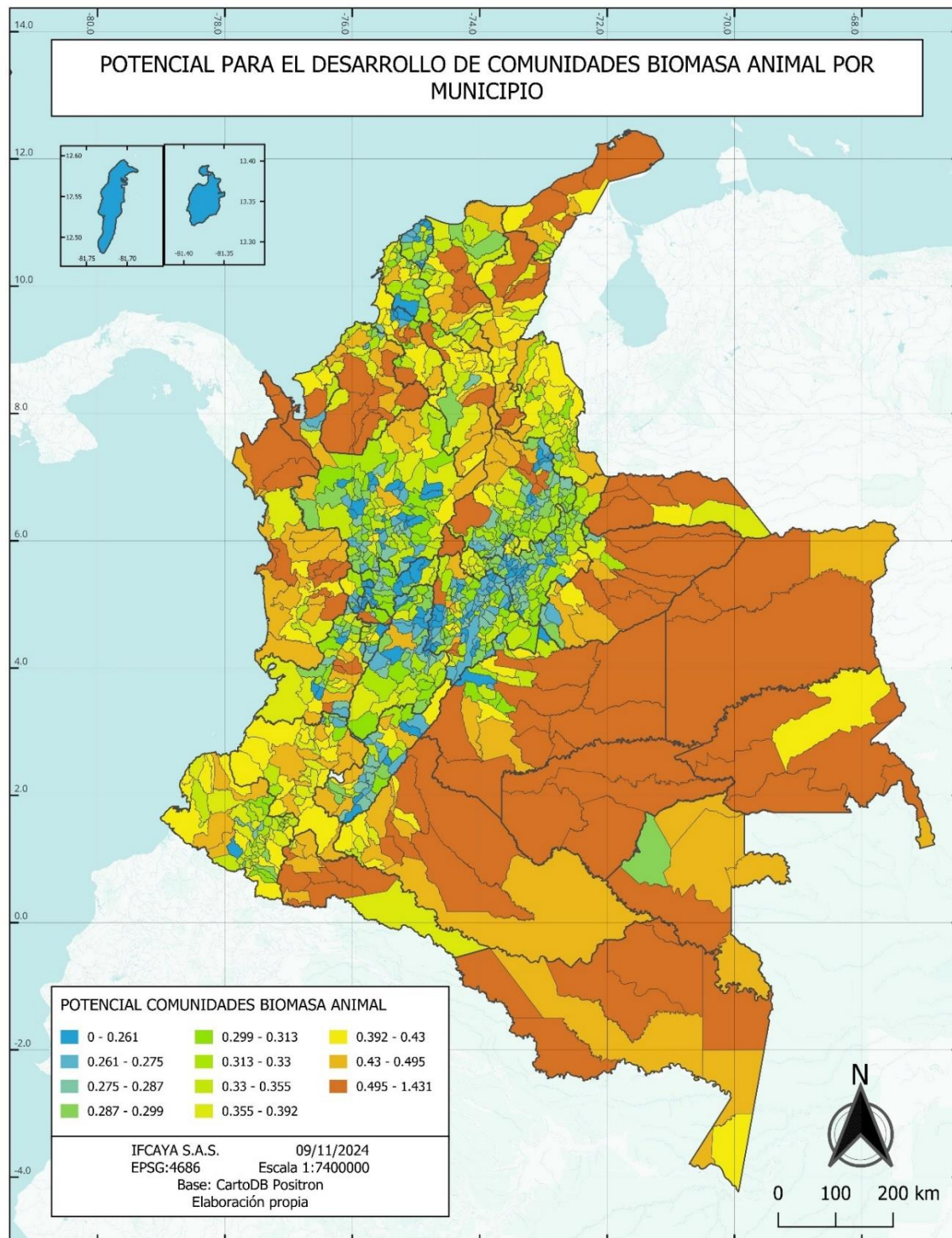
Figura 9. Potencial para el desarrollo de comunidades energéticas - Energía a partir de biomasa animal.
